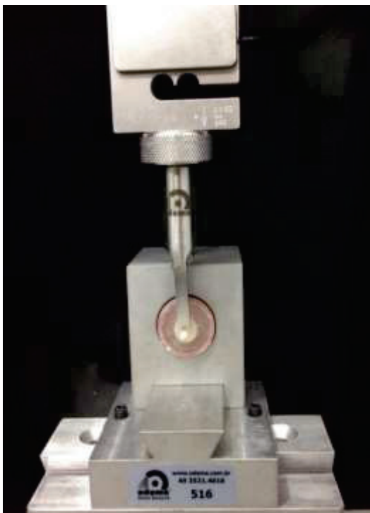
Figura 6: a) Corpo de prova posicionado na máquina de ensaios mecânicos.
