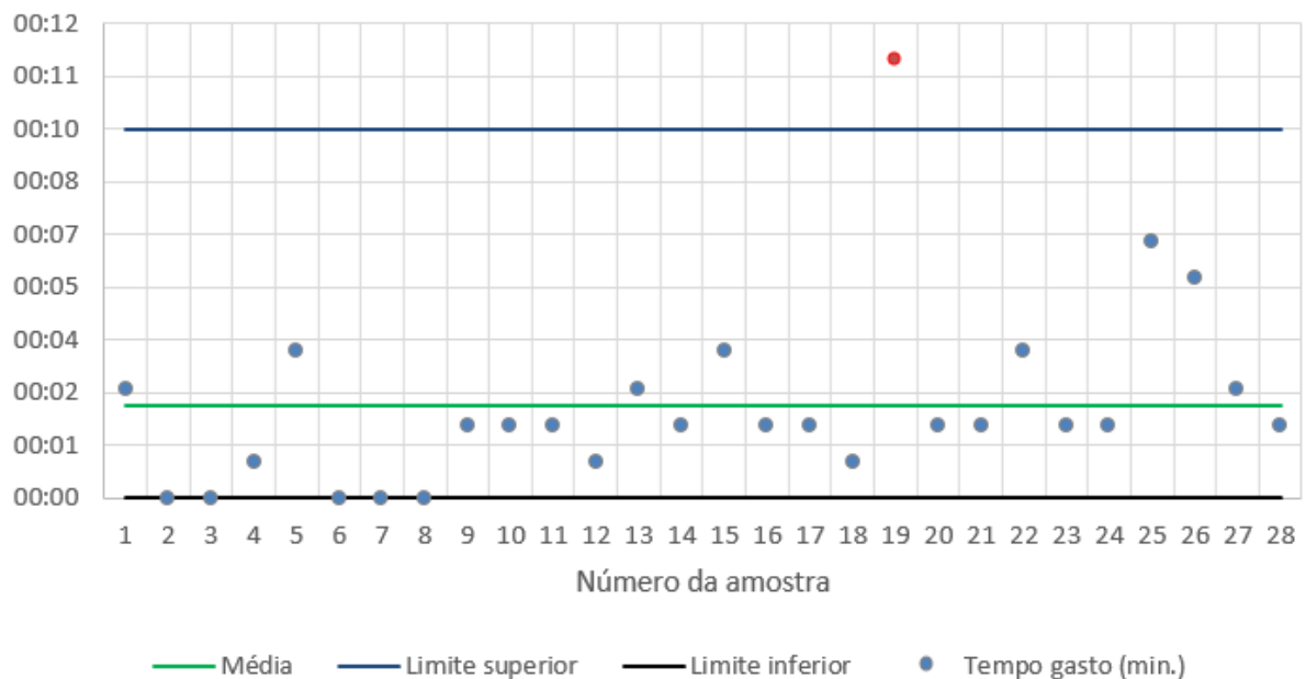
Figura 2 – Gráfico de Controle tempo médio entre chegada e entrada no portão
