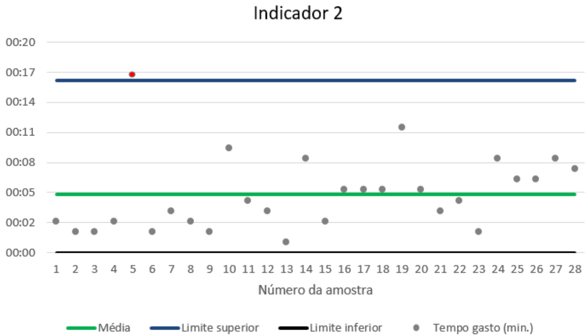
Figura 3 – Gráfico de Controle tempo médio entre entrada no portão e liberação para descarga
