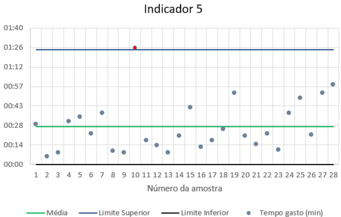
Figura 6 – Gráfico de Controle tempo médio entre chegada e saída do veículo
